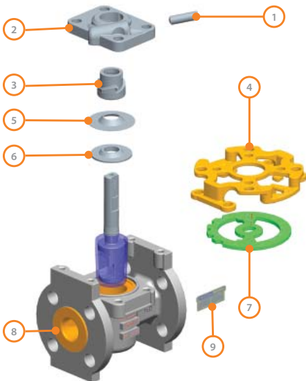
Un éclaté du robinet revêtu
